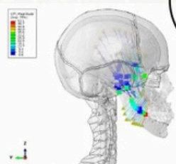
Figura 1. Fuerzas ejercidas músculos y tendones
