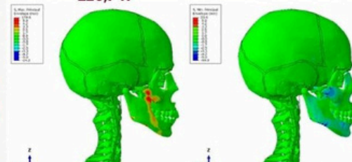
Figura 4. Principales zonas de estrés/menores zonas de estrés [N/mm2]
